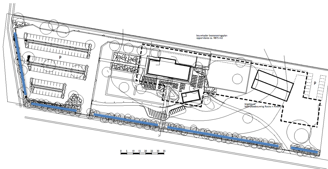
Afbeelding 17. Locatie infiltratiegreppels.
