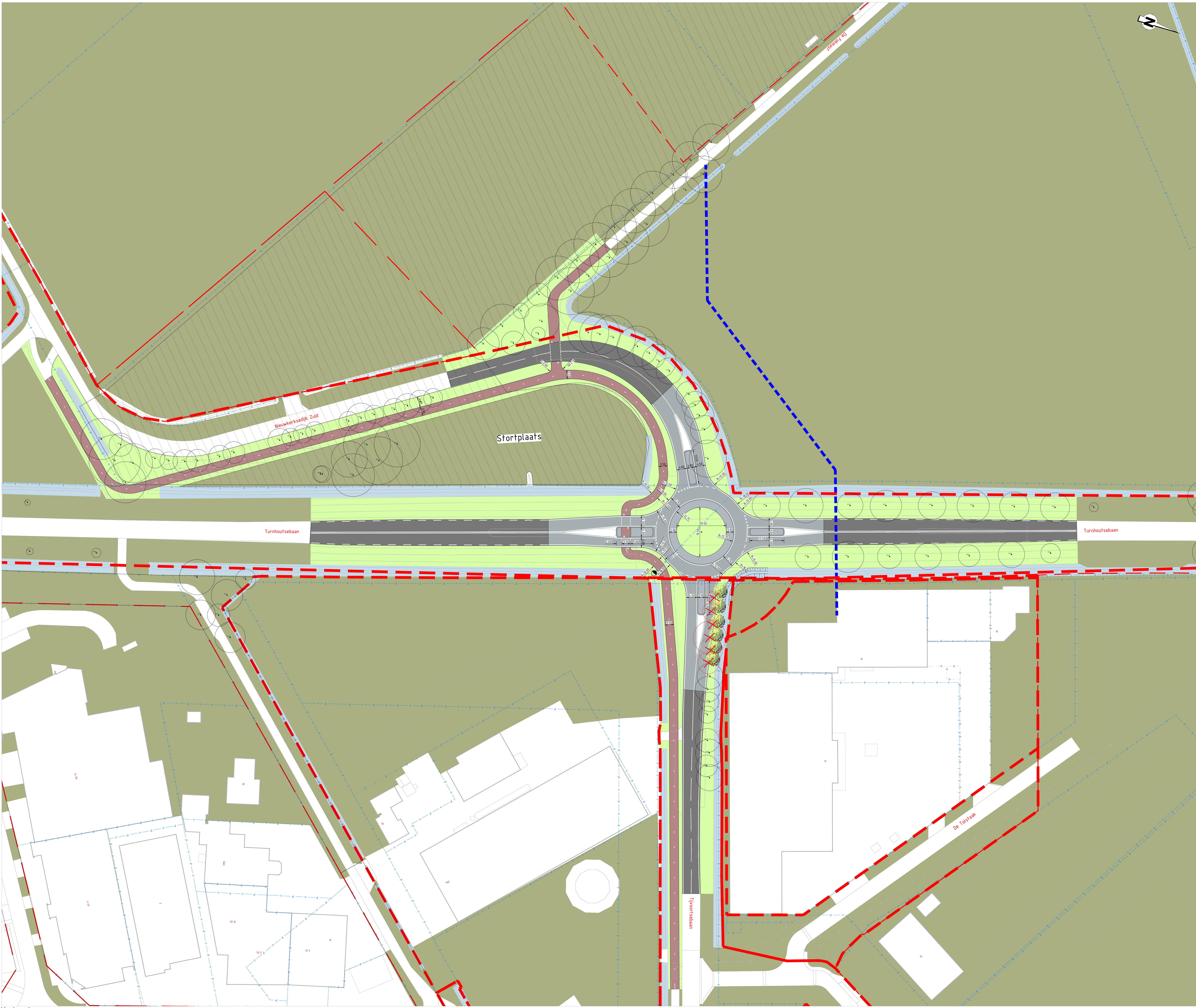
Situatieoverzicht SCHAAL 1 : 5.000
